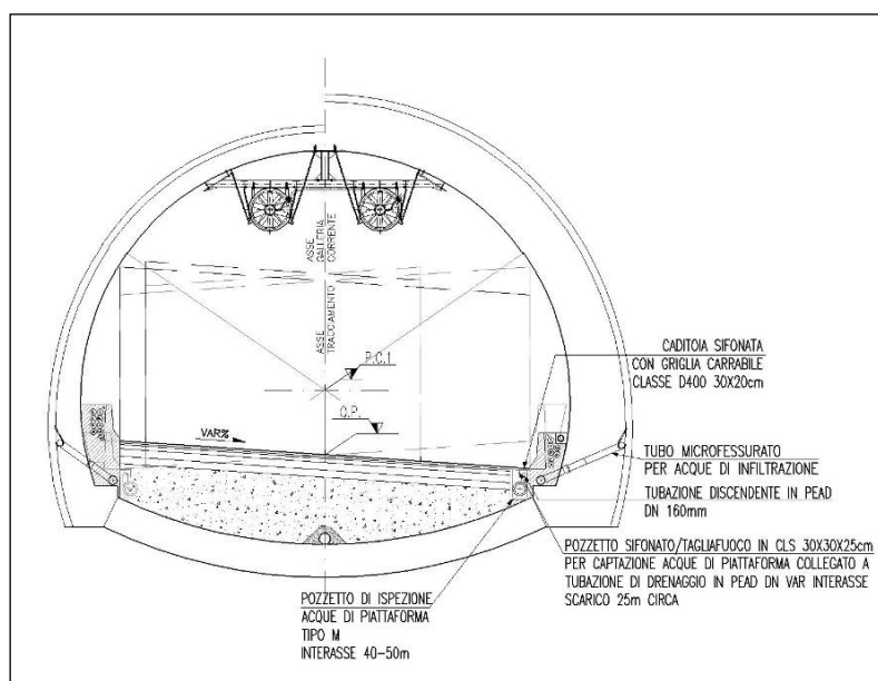
Figura 8.4 - Galleria stradale – Particolare delle opere di drenaggio.
