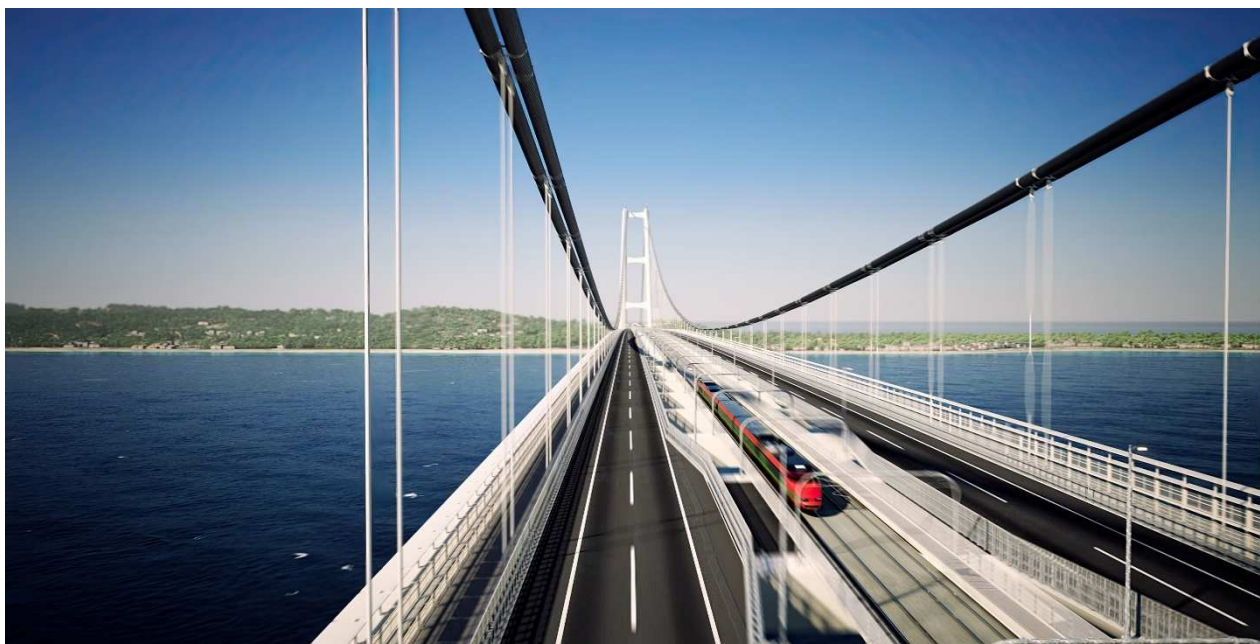
Figura 3.3 - La sezione del nuovo ponte sospeso, esternamente le carreggiate stradali, al centro i binari ferroviari
