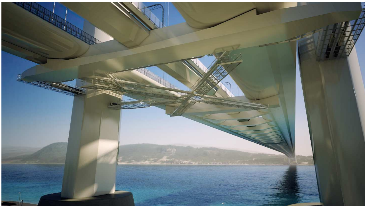
Figura 3.4 - Vista dal basso dell'impalcato in corrispondenza della torre con evidenza dei percorsi per l'ispezione e la manutenzione degli elementi strutturali
